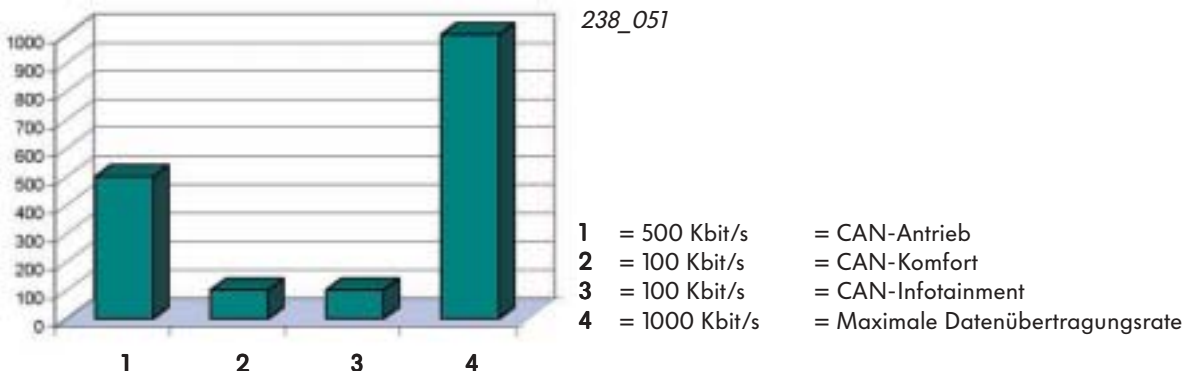
Datenübertragungsraten auf dem CAN-Bus-System
