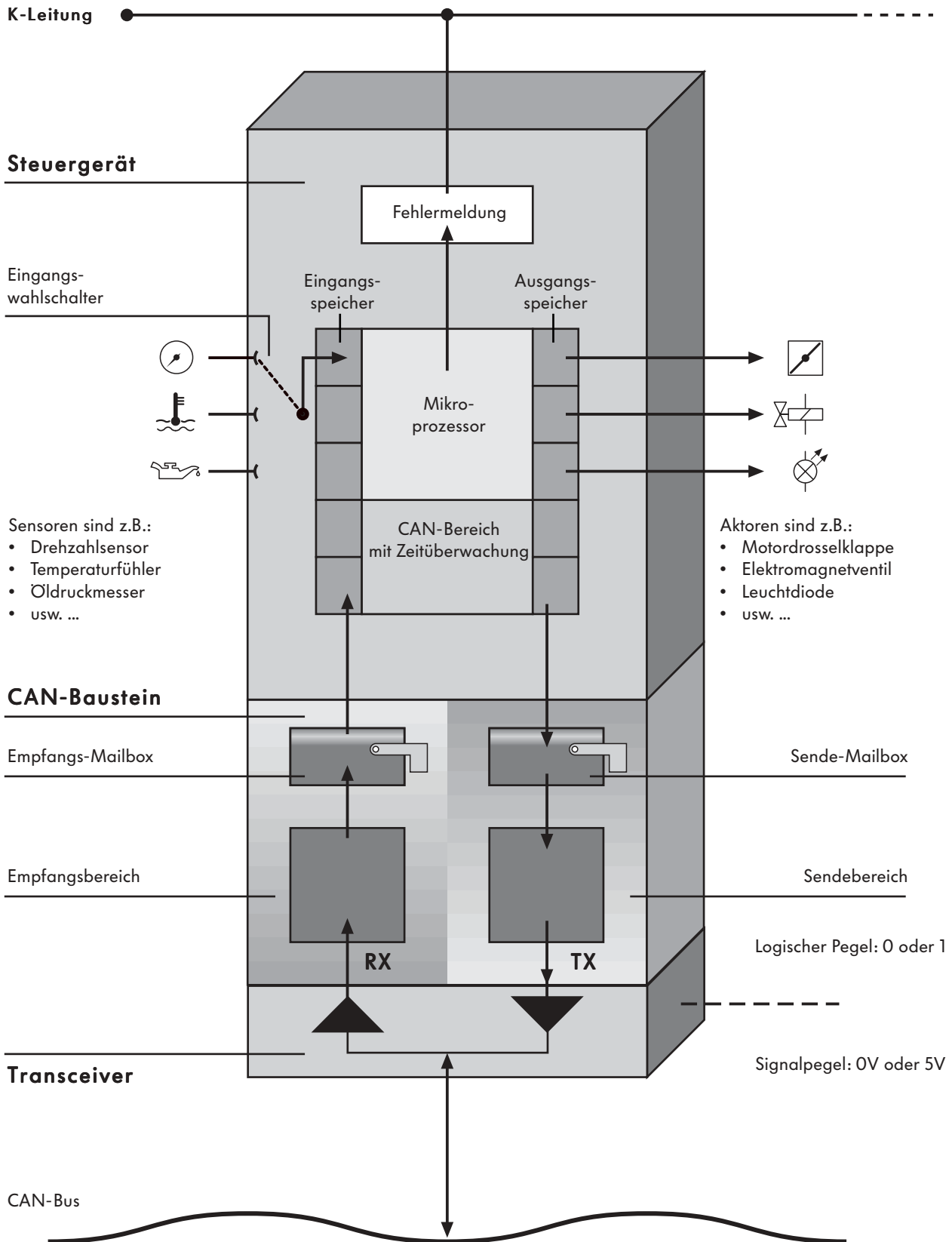
Funktionseinheiten: Steuergerät, CAN-Baustein und Transceiver
