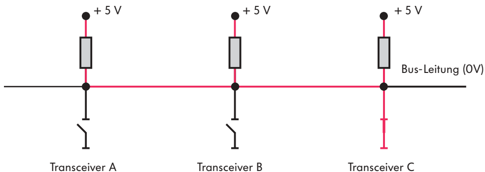
Ankopplung von 3 Transceivern an Bus-Leitung (Prinzip), Transceiver C aktiv
